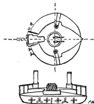
Панцерник берегової оборони „Київ“ (Збуд. 1875, мав 3,350 тонн, 8 вузлів, 2 гармати в 305 мм і панцер від 406 до 460 мм.)
