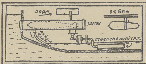
Мал. 2. Підводний мінний апарат (в розрізці).
