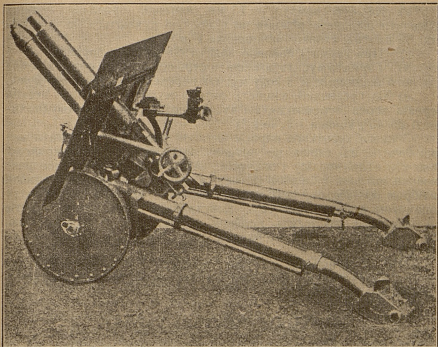
Мал. 4. Англійська 47 мм. піхотна гармата Вікєрса. (рід пушко-гавбвиі).
