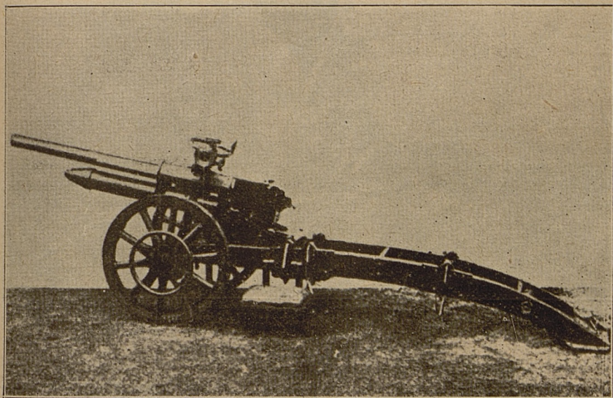
Мал. 2. Англійська 44—60 мм. піхотна гармата Вікерса. (Вигляд гармати з 44 мм. пушечною цівкою).
