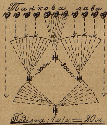
Схема 1. Протитанкова батарея (4 гарм.) в бойовому ладі.
