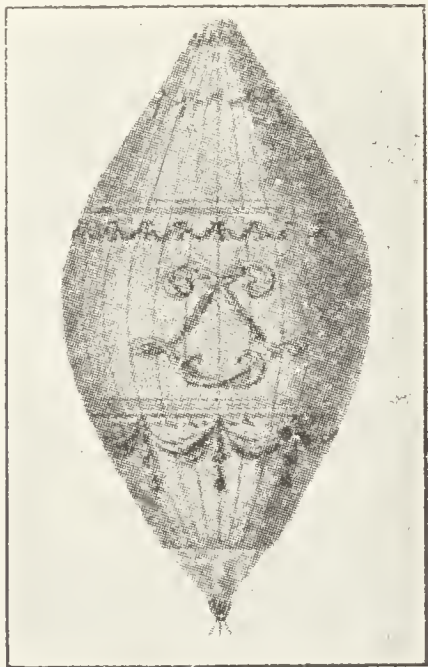
— Перший баллон Монгольф'єра, збудований року 1783 го з полотна а виклеаний папером. Під баллоном був отвір а в ній поміщено посуду, в якій тїла вогня і вогка солюма. Воздух в баллоні поступово грївав ся, а коли теплий воздух виповнив весь баллон, той летів в гору.
