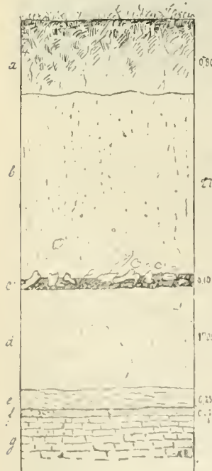
6. Разрѣзъ обрыва въ Мизніи.
