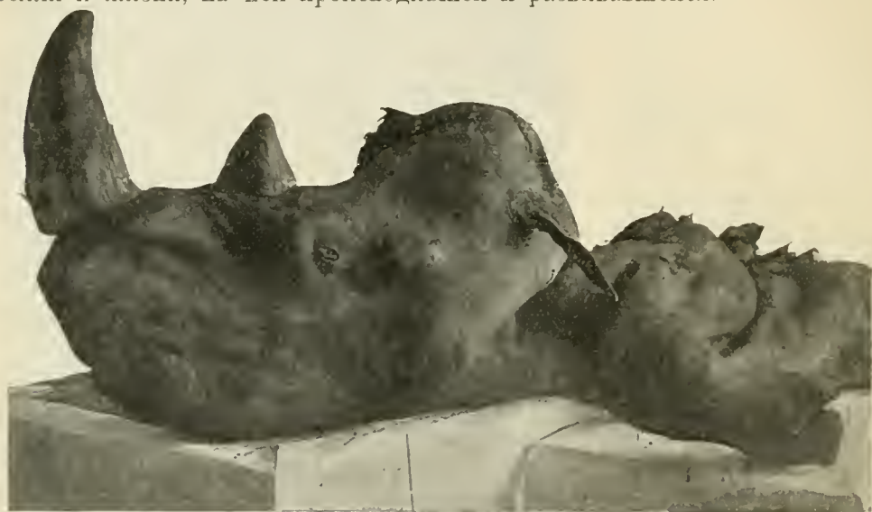
4. Голова диллювіальнаго носорога, выкопанная въ селѣ Старунѣ на галицкомъ Подкарпатѣ
