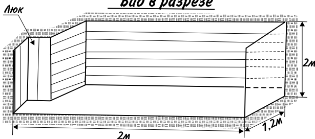
Вид в разрезе
