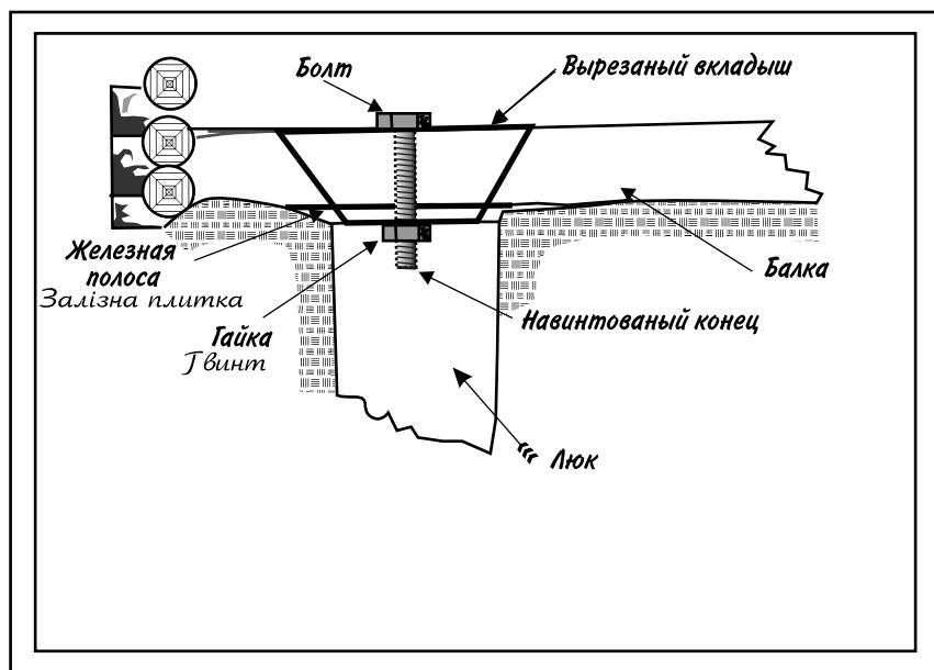
Система крепления крышки люка
