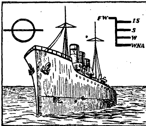
Мал. 2. Грузова марка на борту корабля. Позначення марок роблять на рівні ватерлінії. Для виразності їх показано також окремо у збільшеному вигляді. Значення літер пояснено в тексті
