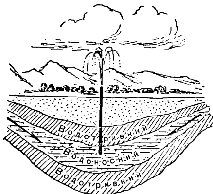
Розріз артезіанського колодязя.
