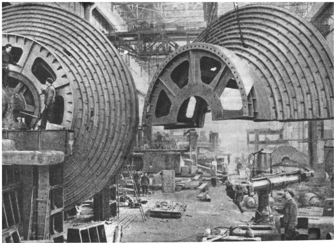
Завод підоймальних машин у Краматорську.
