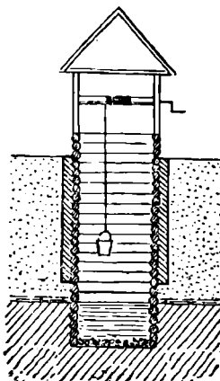
Розріз колодязя.
