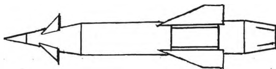
Рис. ч. 4. ASM-N. 7A. BULLPUP ЗДА. Довжина 10 стіп і 6 інчів, об'єм 3 стопи і 1 інч. Вага 570 фунтів.
