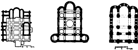
Поземні плани церков: Десятинної в Києві, Спасо-Преображенської в Чернігові й Кирилівської в Києві.
