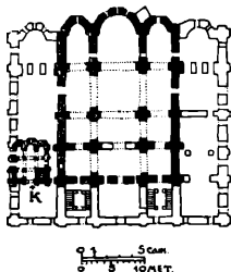
Поземний план Успенської Лаври. Грубими лініями позначене первісне заложення, тонкими — пізніші добудови.
